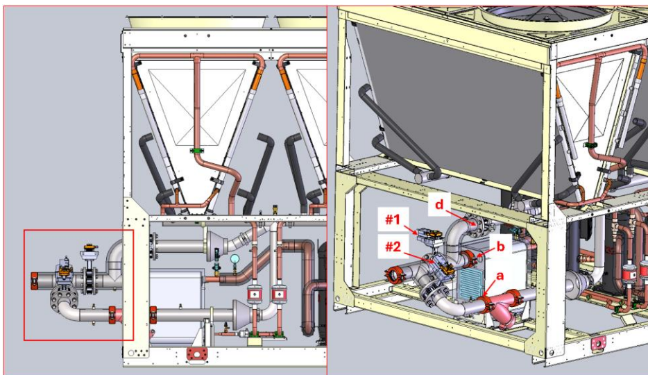
Joonis 19- Torustiku paigaldamise üksikasjad.
