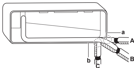
A Vasakpoolne torustik B Vasakpoolne tagaosas torustik C Vasakpoolne allosa torustik a Eemaldage siit toruava sisendi kate vasakpoolse torustiku jaoks b Eemaldage siit toruava sisendi kate vasakpoolse allosa torustiku jaoks
