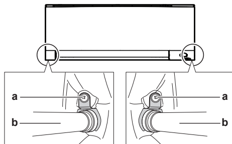
a Isolatsiooni kinnituskruvi b Drenimisvoolik
